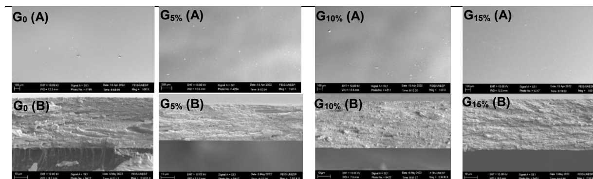
Figura 3 - Micrografias de superfície (A) e de fratura mecânica (B) dos filmes puro e nanocompósitos a base de gelatina Fonte: autoria própria
